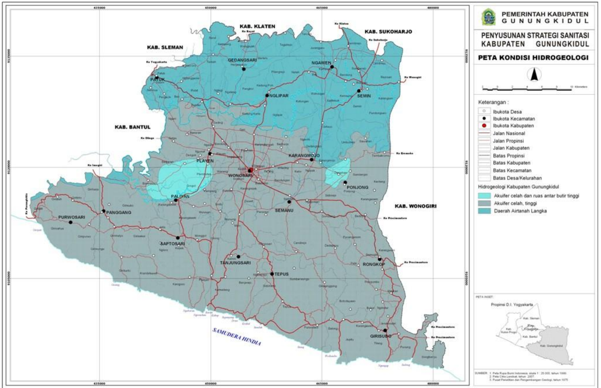
Peta Kondisi Hidrogeologi Sumber : Bappeda Kab. Gunungkidul
