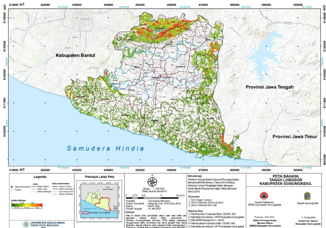
Gambar 3.10 Peta Bahaya Tanah Longsor di Kabupaten Gunungkidul
